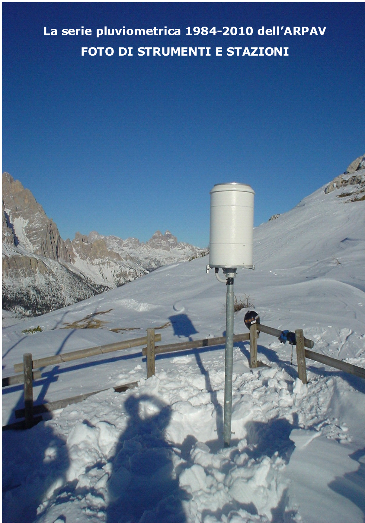
Pluviometro MTX con bocca da 1000 cm 2 della stazione ARPAV del Monte Faloria.
