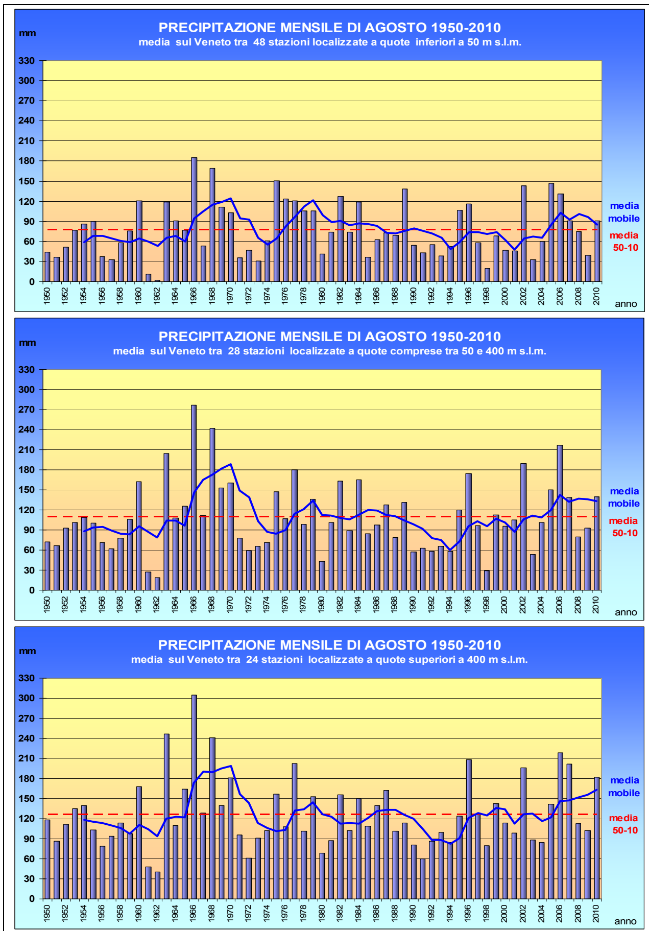
Fig. 57 - Precipitazioni del mese di agosto nel periodo 1950-2010 (media zonale).
