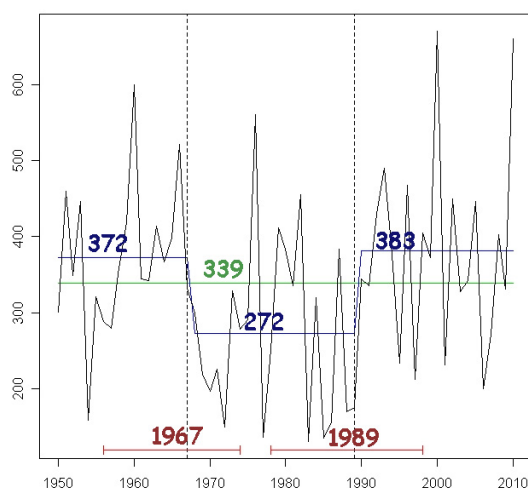
Fig. 84 - Precipitazione autunnale media e breakpoints calcolati sui valori medi/annui di tutte le stazioni Dalla analisi della figura 84 si evidenzia:
