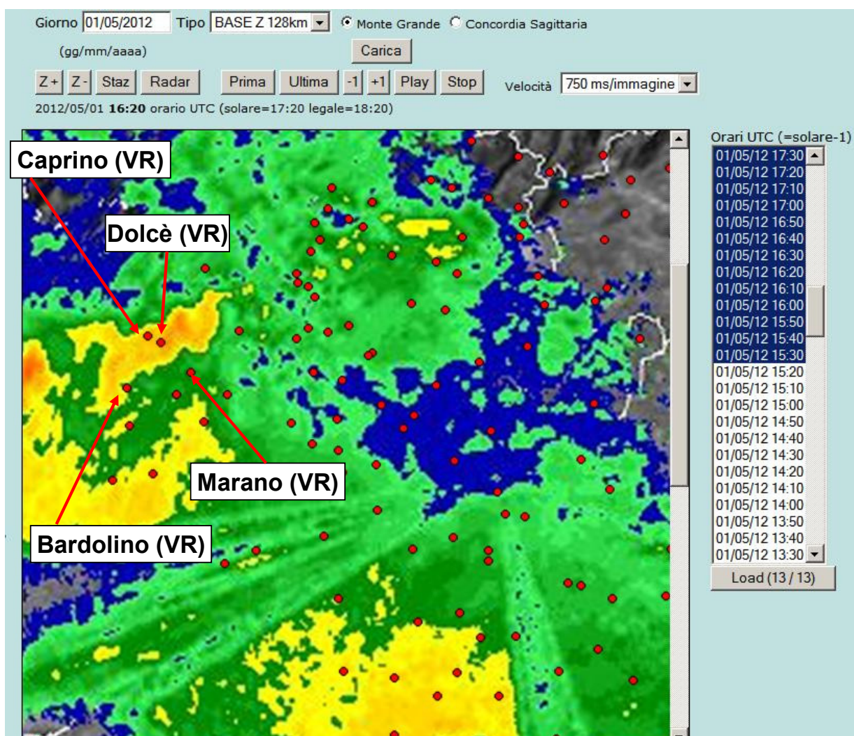
Fig.23 – I dati radar delle ore 17.20 solari del 1 maggio 2012 spiegano la diversa intensità di precipitazione rilevata dalle 4 stazioni del grafico sopra riportato.
