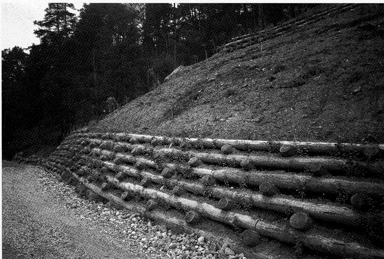
Foto n. 1 - Palificata in legname con messa a dimora di piantine (al termine della fase di costruzione) (San Genesio - Bz) Tipologia n. 14
