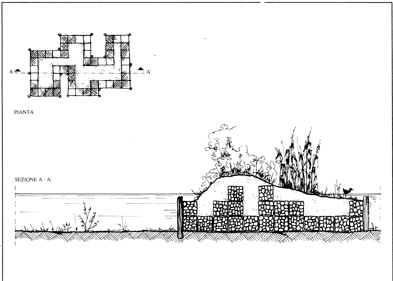
Fig. 21 - Isola in gabbioni ricoperta di terreno ed inerbita
