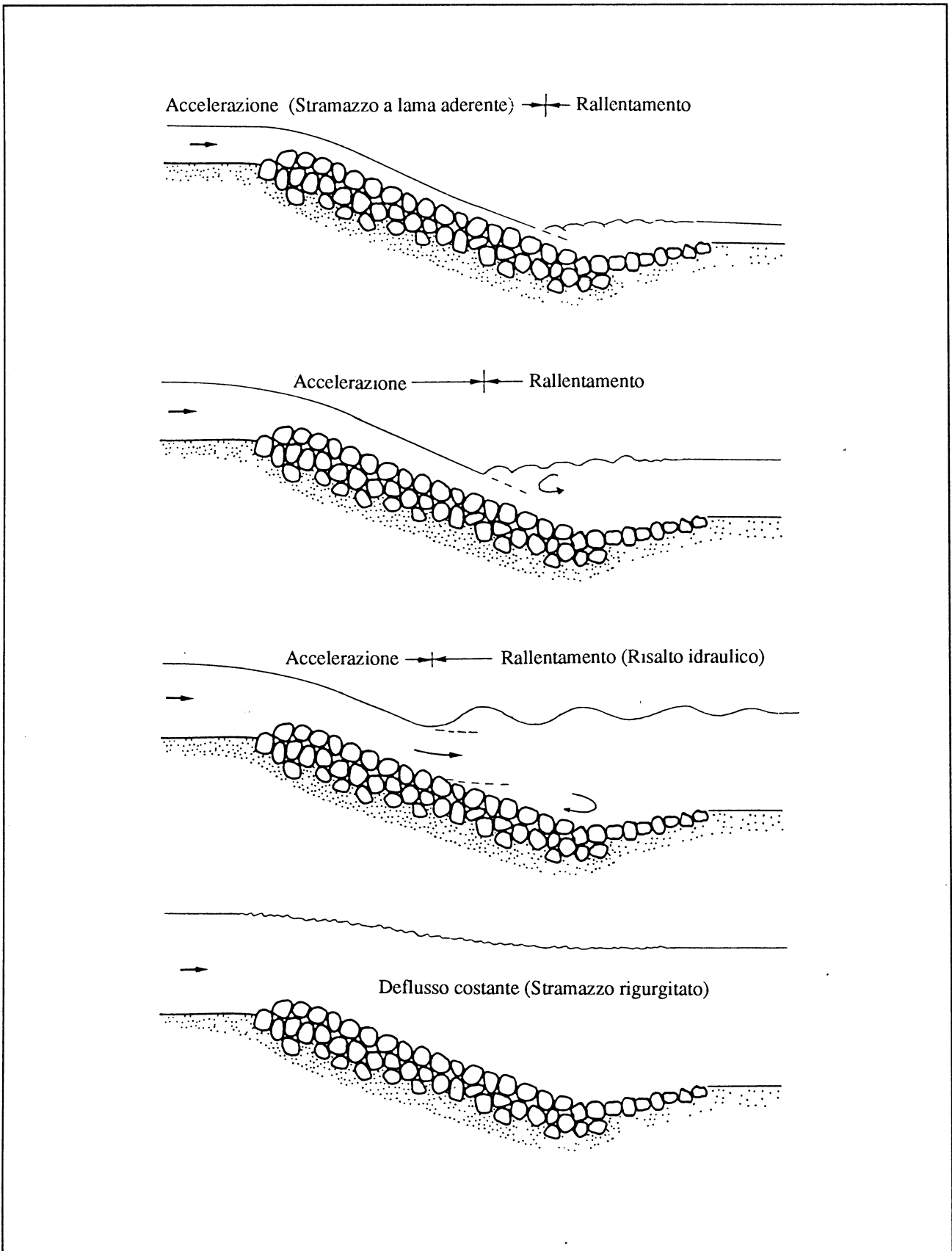
Fig. 41 - Aspetti fluido-dinamici della corrente in funzione di portate idriche crescenti (Gebler, 1990)
