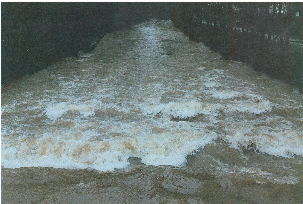
TAV. N. 35 Rampa in pietrame (portata di piena di 20 mc/sec) (Fiume Odenwulder Elz) Tipologia n. 26 a8
